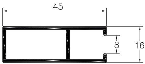
CB.41 Lateral Móvel
