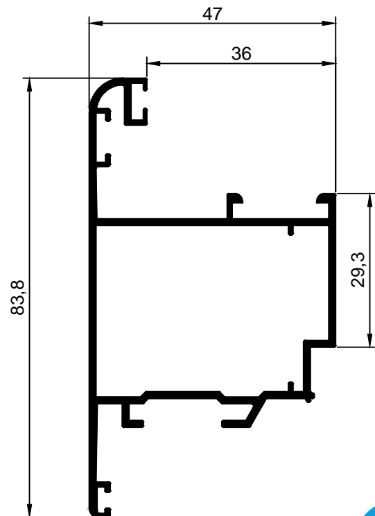
AQ.33 Aro Móvel Abt. Exterior
