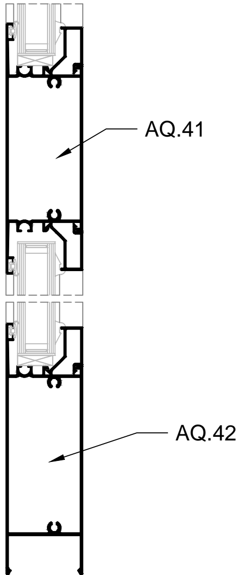
corte vertical escala: 1/2
