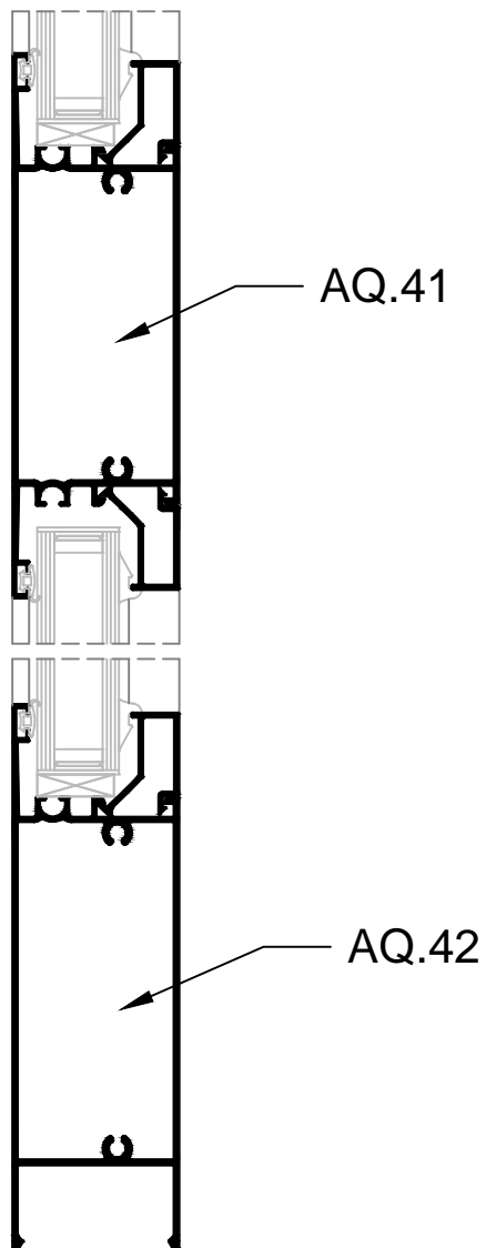
corte vertical escala: 1/2
