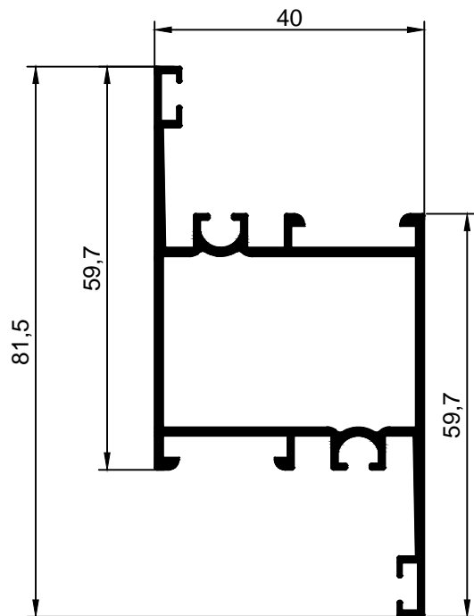
AQ.16 Travessa Inversora
