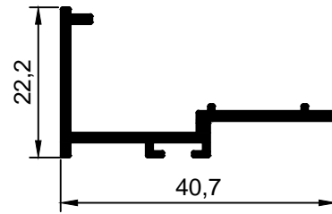
AQ.86 Bite Vedação Inferior
