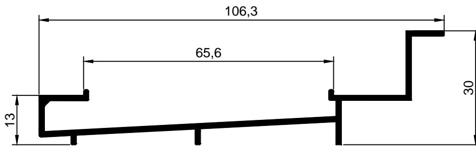
AQ.82 Soleira Condensação
