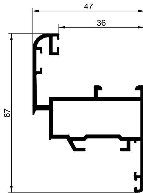
AQ.21 Aro Móvel
