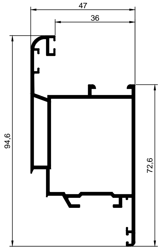
AQ.35 Aro Móvel
