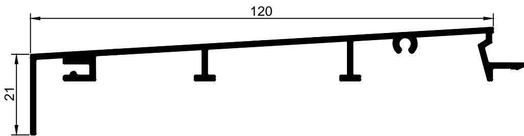
AQ.116 Esquadro P/ST.83
