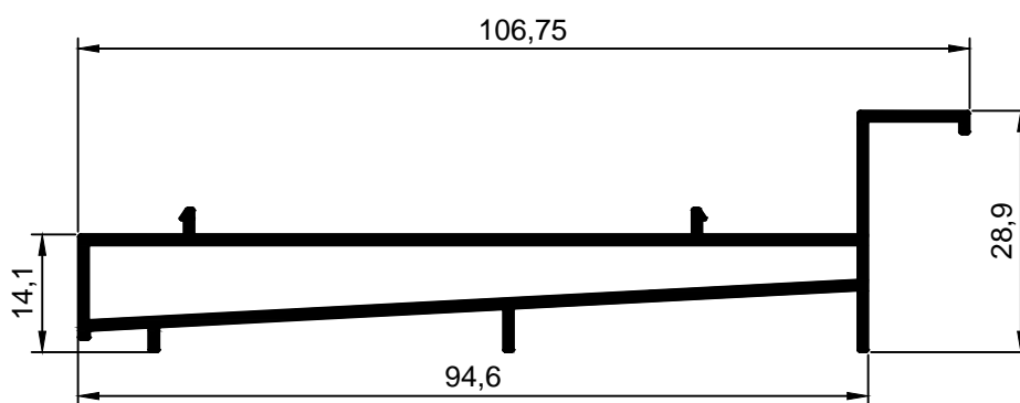
AQ.89 Soleira Condensação
