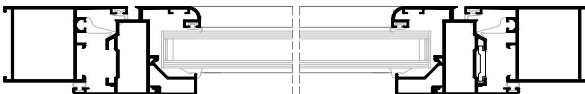
corte horizontal escala: 1/2
